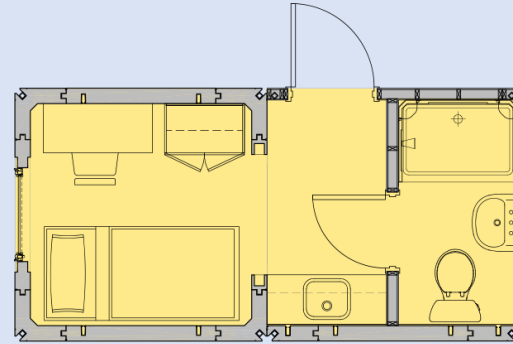
2 MODULE INTERIM UNIT
